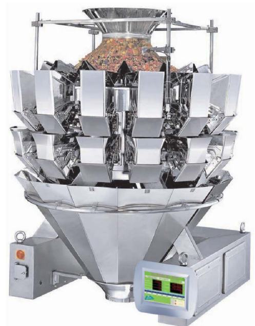
DW-MH/C14/25 Pesadora Multicabezal Circular de 14 básculas y 2.5 l de capacidad
